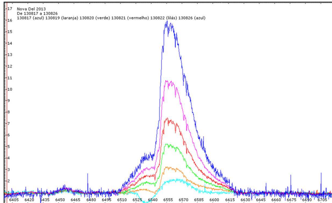
Nova Delphini 2013 entre 130817 e 130826
