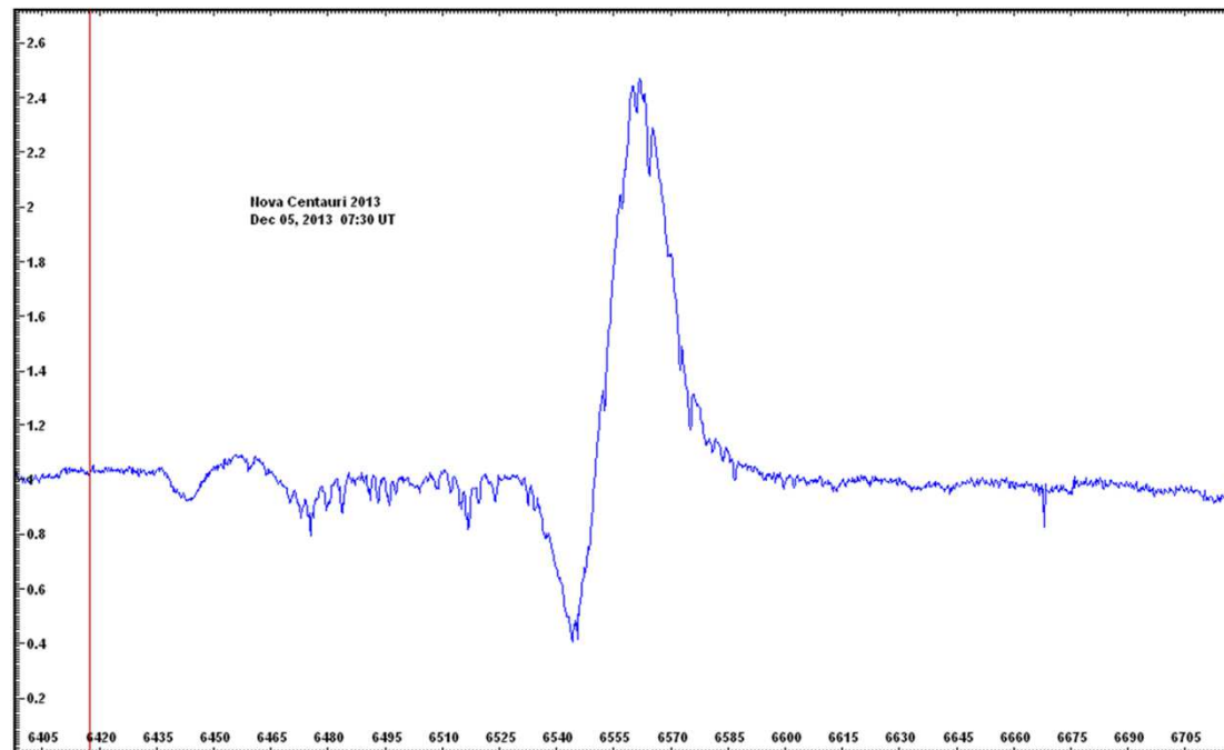
H-Alfa na Nova Centauri 2013 (20131205)
